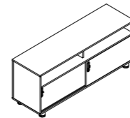
Armário baixo *com 02 portas de correr *02 nichos superiores ORD1605 - 1600 X 472 X 625
