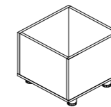
Container *01 lugar ORD4703 - 472 X 472 X 432
