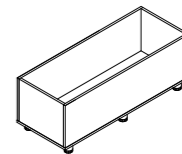
Container *03 lugares ORD1233 - 1200 X 472 X 432
