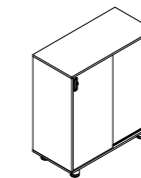
Armário médio *com 01 porta de correr *com 02 prateleiras móveis
