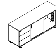
Armário baixo *com porta de correr *com gaveteiro e nicho para CPU ORD1609 - 1600 X 472 X 625
