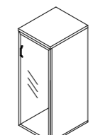
Armário médio *02 prateleiras móveis *porta de vidro fumê 4mm
