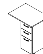
Gaveteiro lateral *com extensão *com 02 gavetas e 01 gavetão *com 01 fechadura
