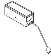
Caixa de tomada *com tomadas elétricas e plug ACT3016 - 300 X 135 X 145
