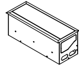
Caixa de tomada *com tomadas elétricas ACT3015 - 300 X 135 X 145
