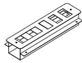
Régua tona *com tomadas elétricas ACT3075 - 294 X 98 X 55
