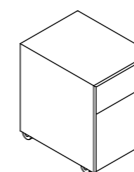
Gaveteiro Móvel *01 gaveta e 01 gavetão GPL6103 - 430 X 550 X 613
